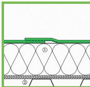
Çizgisel yapıştırma metodu 1) Isı yalıtımı katmanı 2) Altyapı katmanları 3) KÖSTER TPO Sentetik Örtü (yeşil katman)
