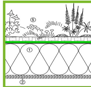
Yeşil çatı teras detayı 1) Isı yalıtımı katmanı 2) Alt yapı katmanları 3) KÖSTER TPO Sentetik Örtü (yeşil katman)
