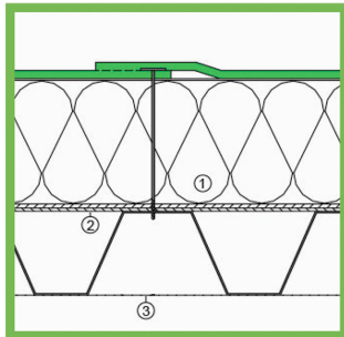
Mekanik tespit metodu 1) Isı yalıtımı katmanı 2) Alt yapı katmanları 3) Trapezoidal metal çatı levhası 4) KÖSTER TPO Sentetik Örtü (yeşil katman)
