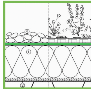
Serbest serme (üzeri balastlı) metodu 1) Isı yalıtımı katmanı 2) Alt yapı katmanları 3) KÖSTER TPO Sentetik Örtü (yeşil katman) 4) Çakıl 5) Yeşil çatı katmanı
